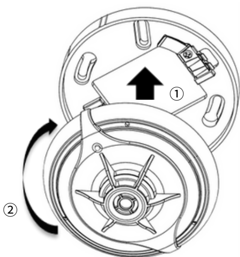
[Hình 5] Cách lắp đầu báo
