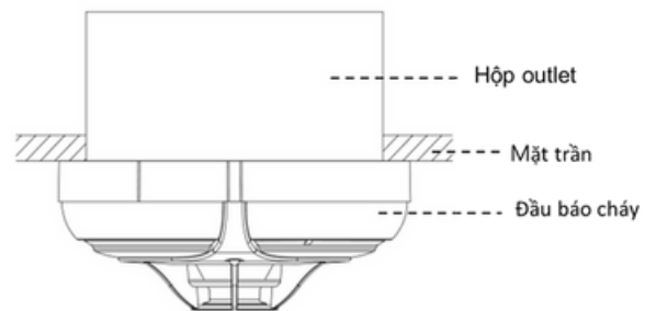
[Hình 1] Ví dụ lắp đặt cho trần đơn.
