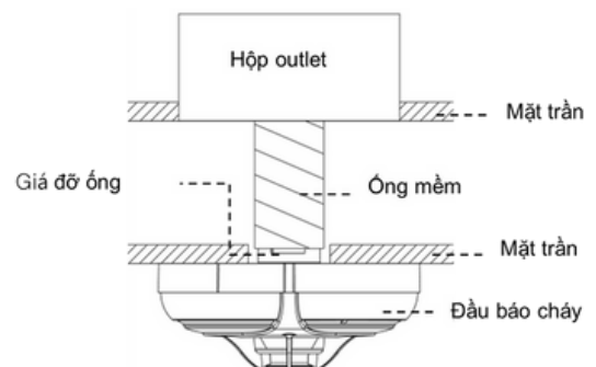
[Hình 2] Ví dụ lắp đặt cho trần đôi.
