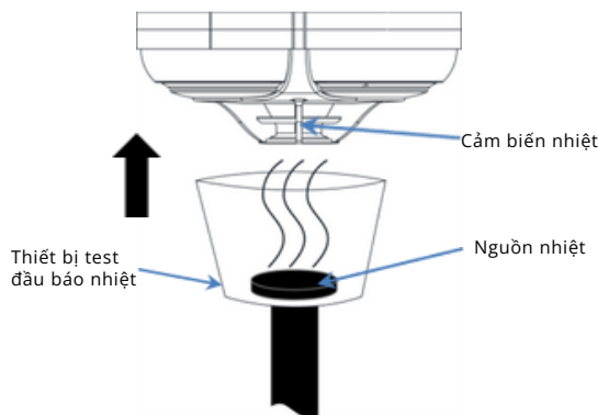
[Hình 10] Test đầu báo nhiệt
