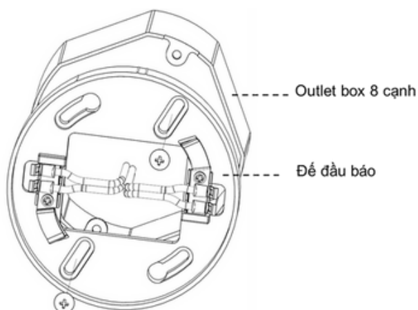
[Hình 4] Outlet Box 8 cạnh
